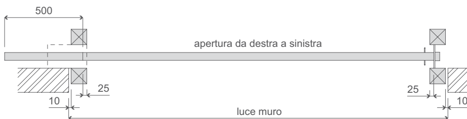
VISTA ESTERNA
