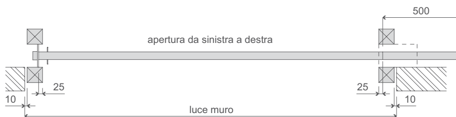
VISTA ESTERNA
