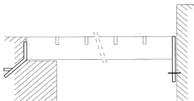
Applicazione di zanche a murare o tassellare
