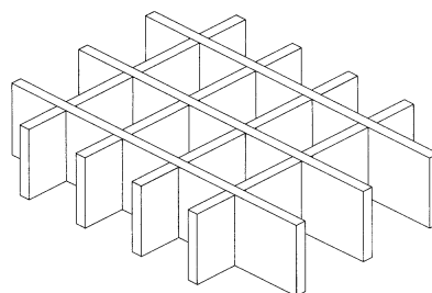
Realizzazione Duplex con piatti di uguale sezione
