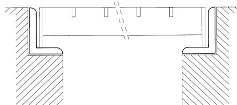
Applicazione del piatto di livellamento
