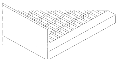
Applicazione del piatto parapiede
